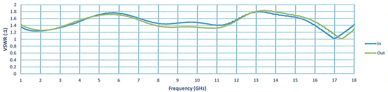
VSWR
