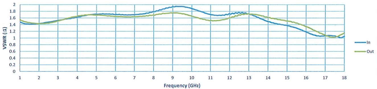
VSWR
