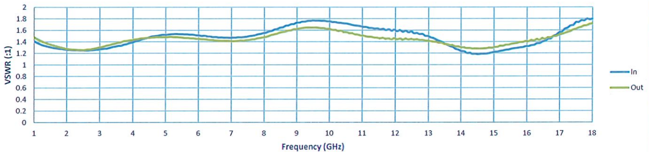
VSWR
