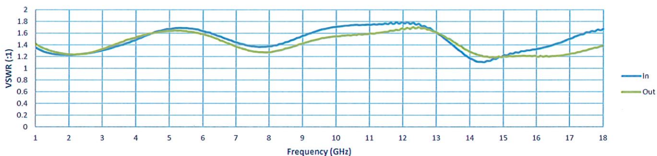
VSWR
