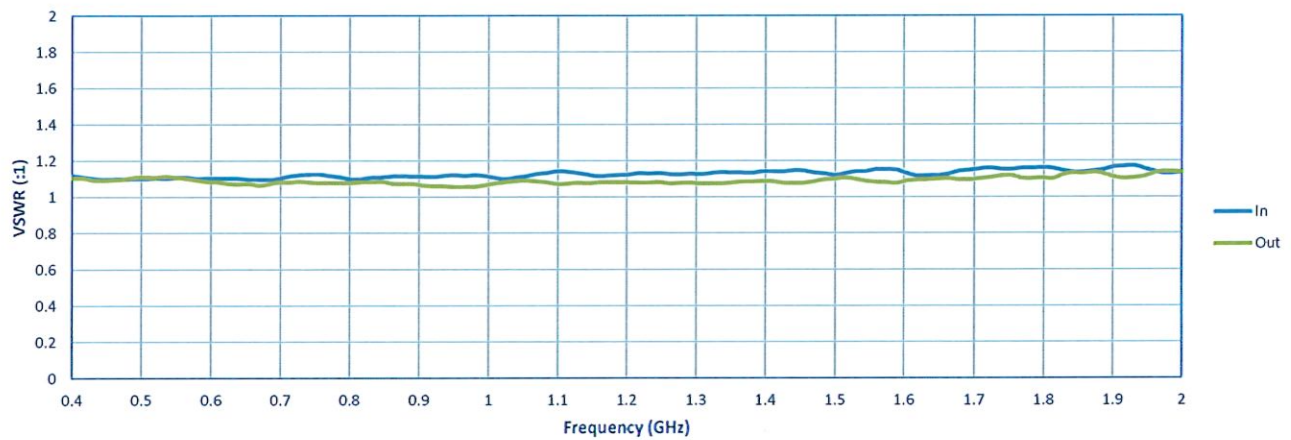
VSWR
