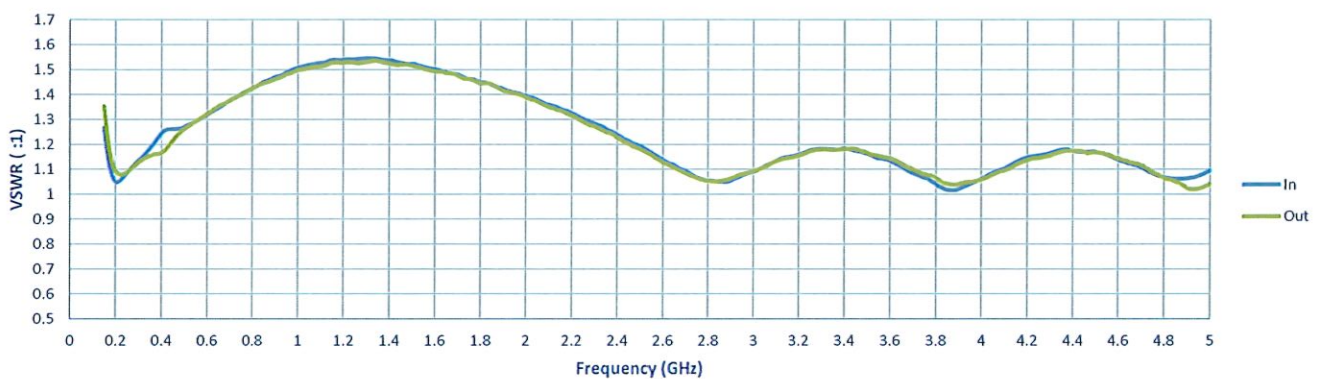
VSWR
