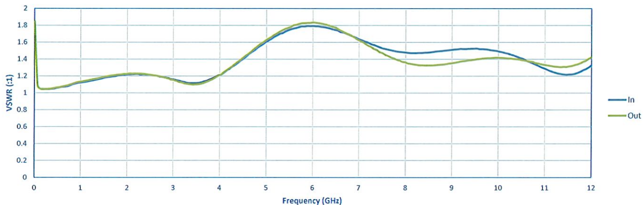
VSWR
