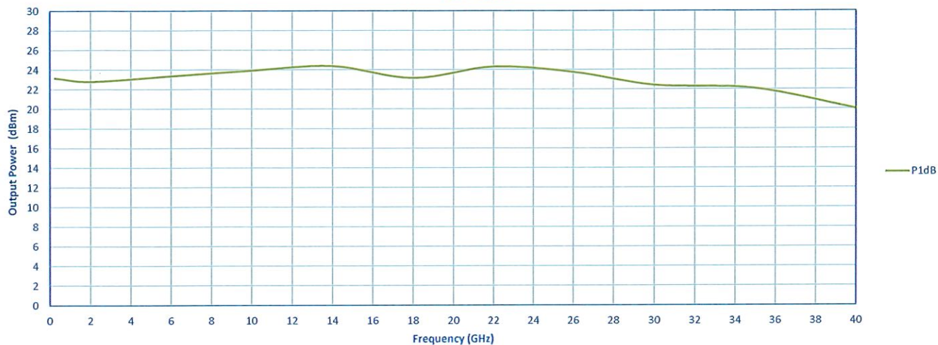
OP1dB
