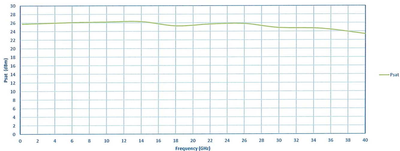
PSAT
