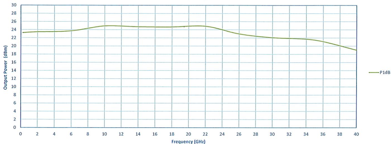
OP1dB
