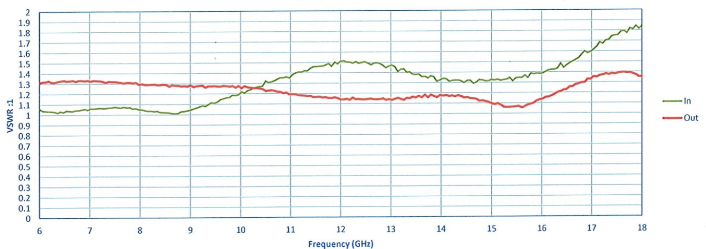
Input/Output VSWR
