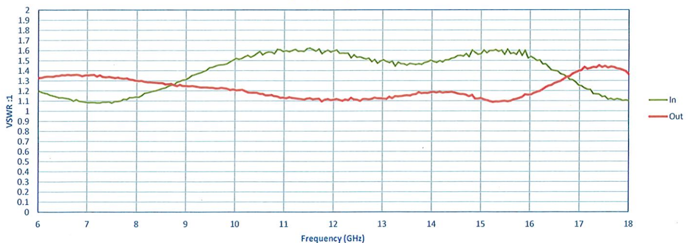
Input/Output VSWR
