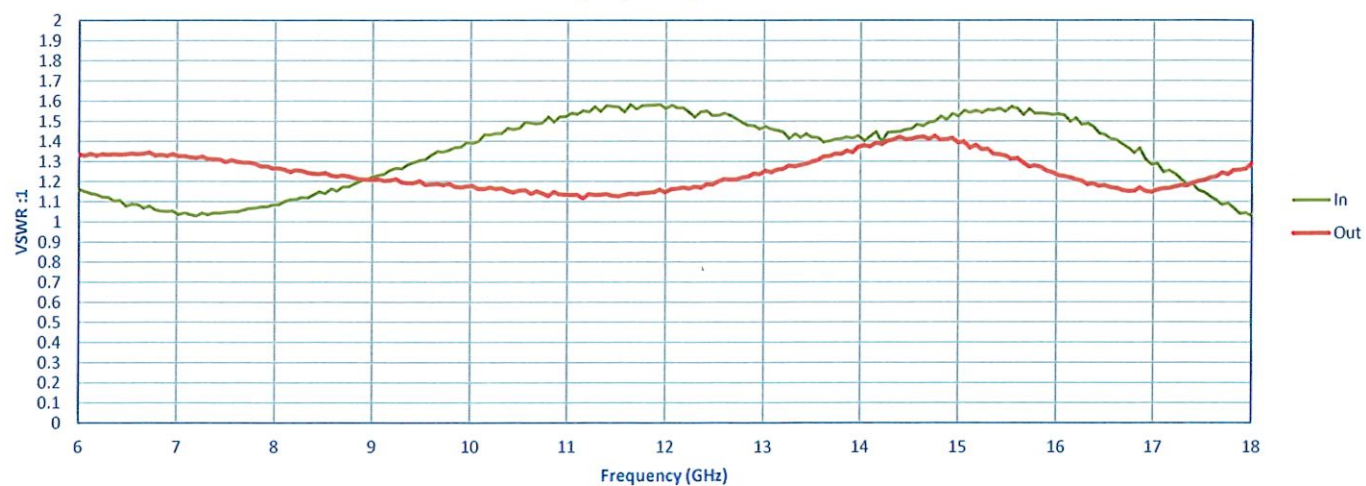
Input/Output VSWR
