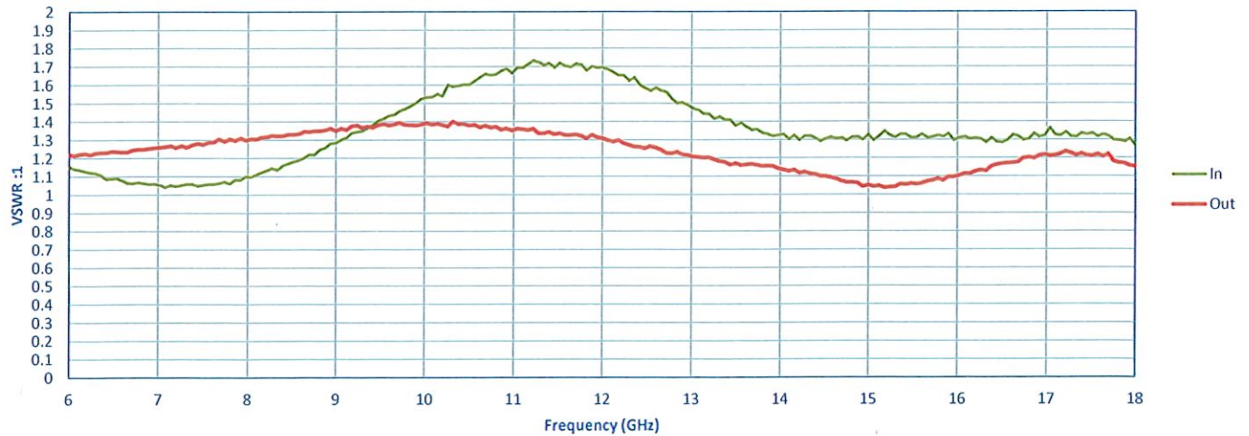
Input/Output VSWR
