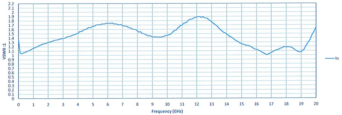
Input VSWR
