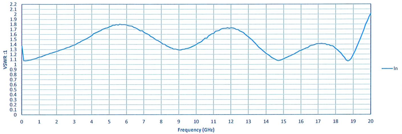
Input VSWR
