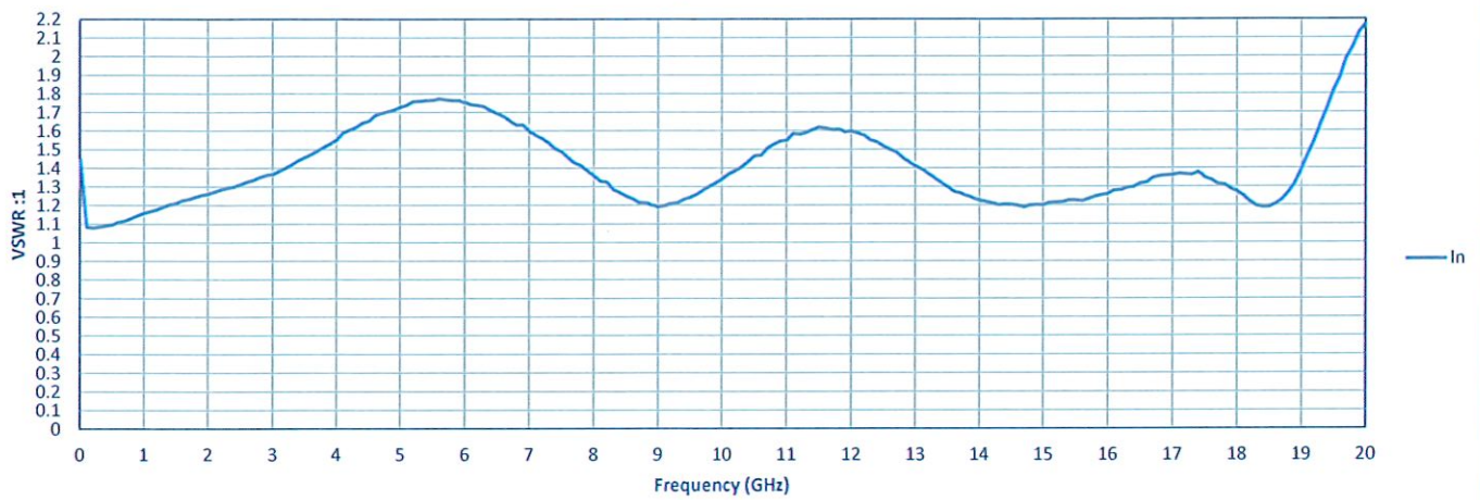
Input VSWR
