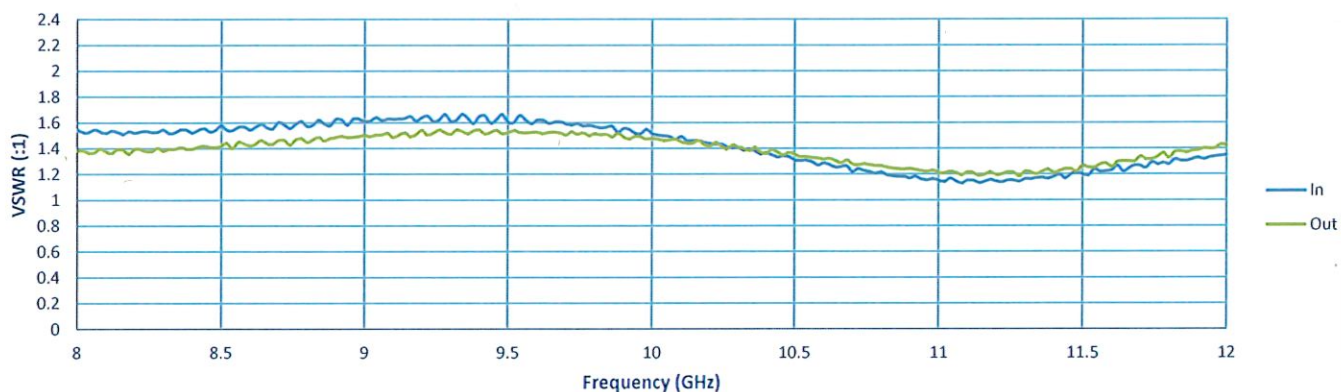
VSWR
