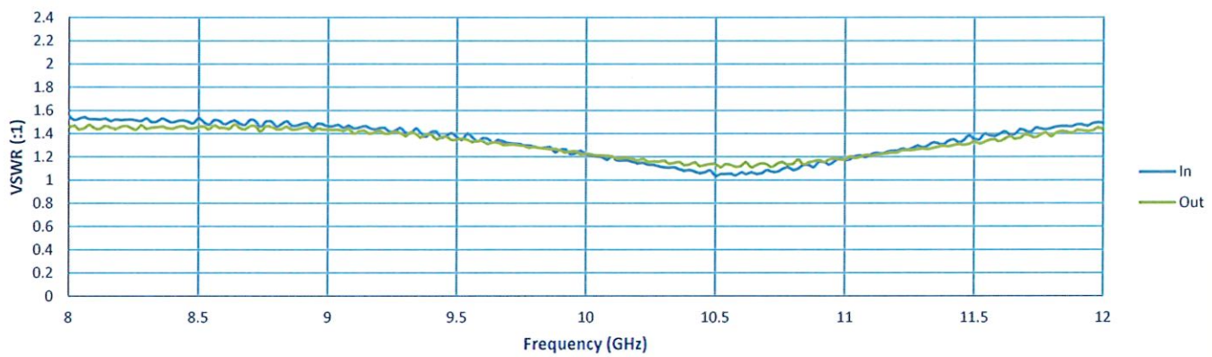
VSWR
