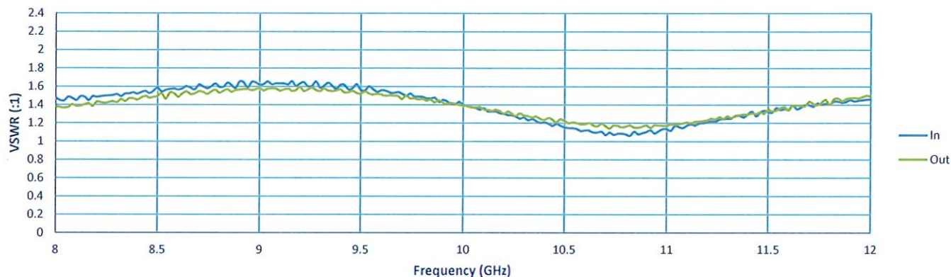
VSWR
