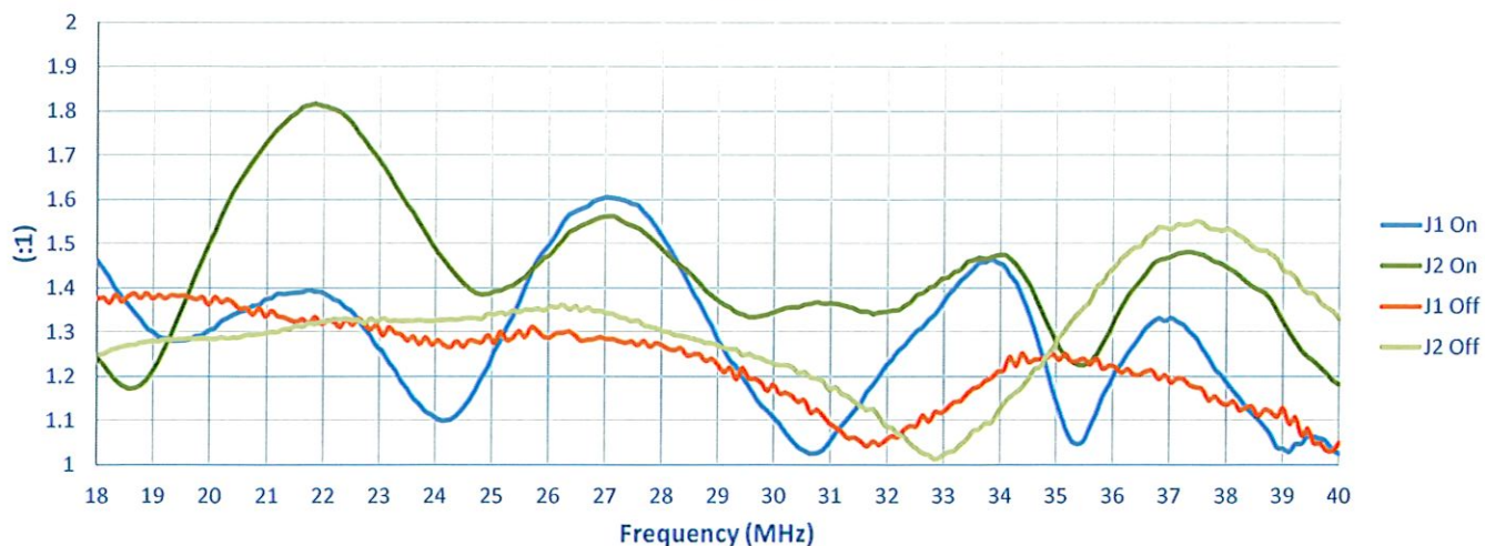
VSWR
