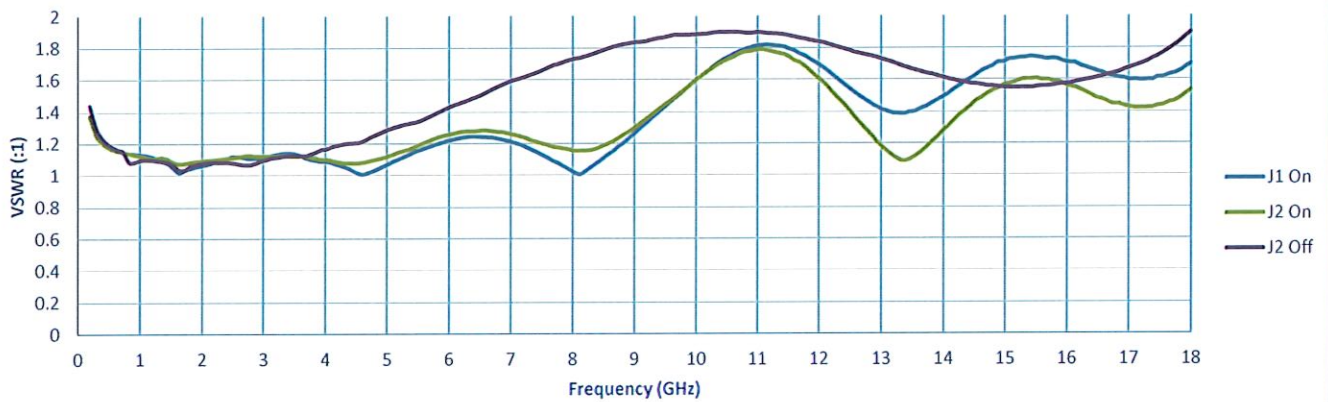
VSWR
