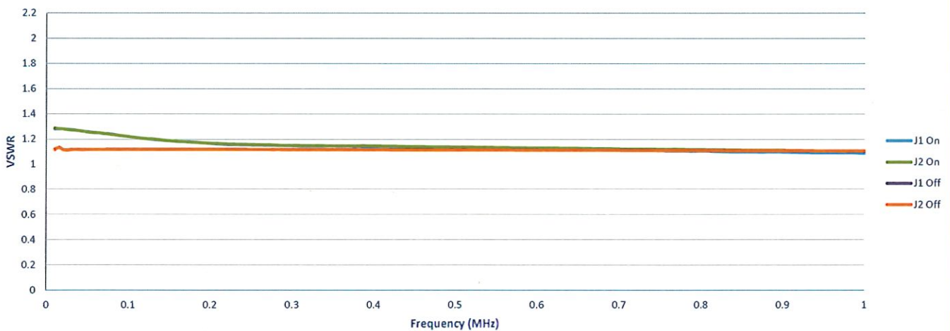
VSWR
