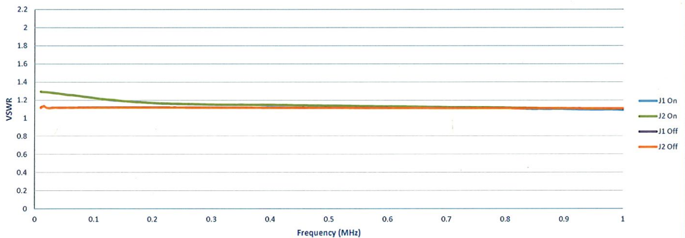
VSWR
