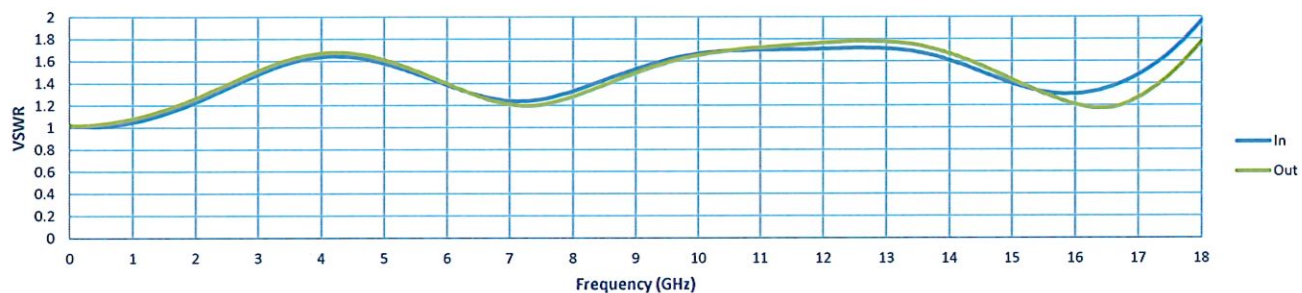
VSWR
