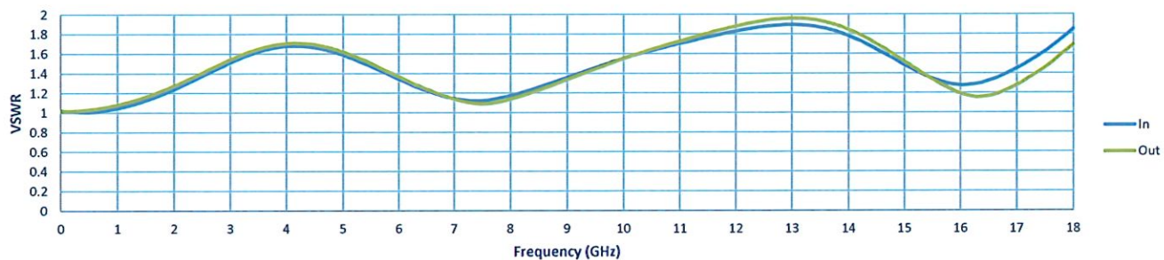
VSWR
