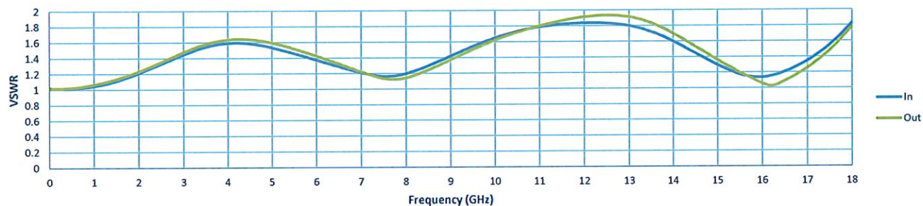
VSWR
