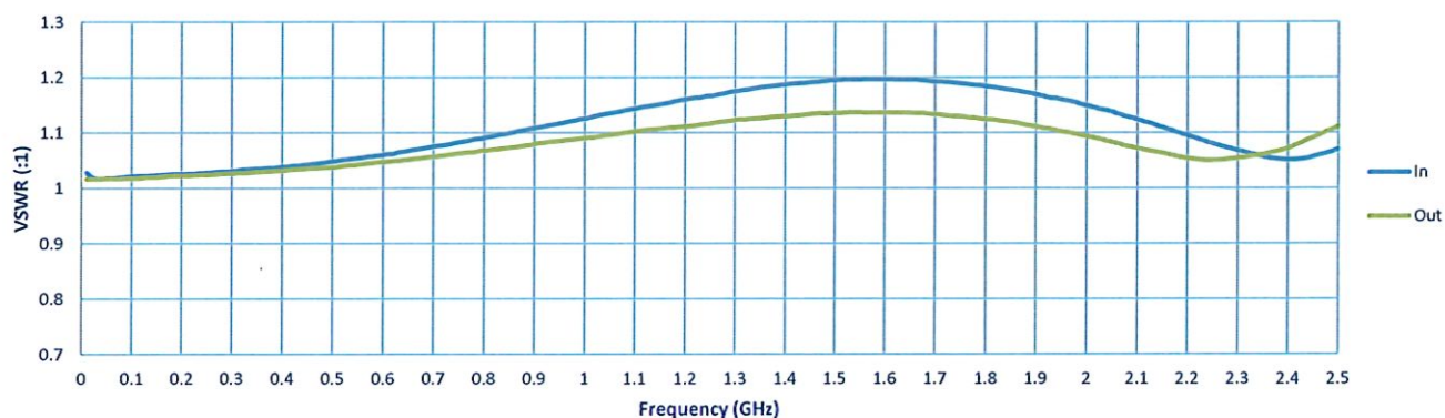
VSWR
