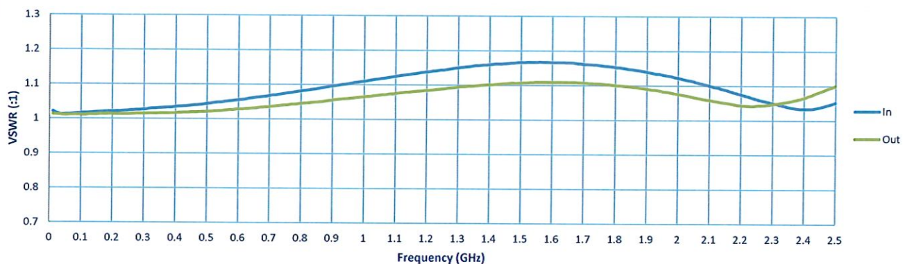
VSWR
