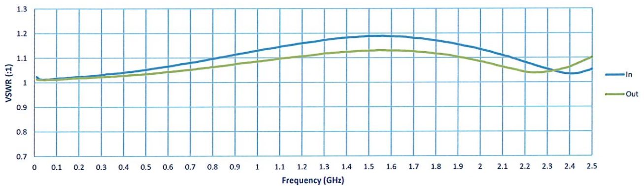
VSWR
