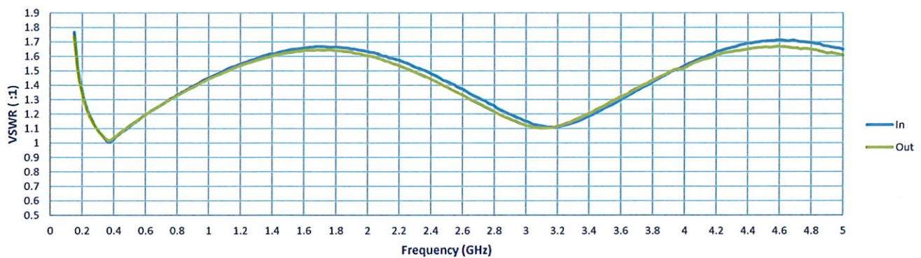
VSWR
