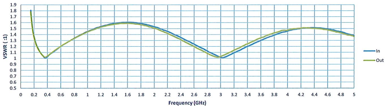
VSWR
