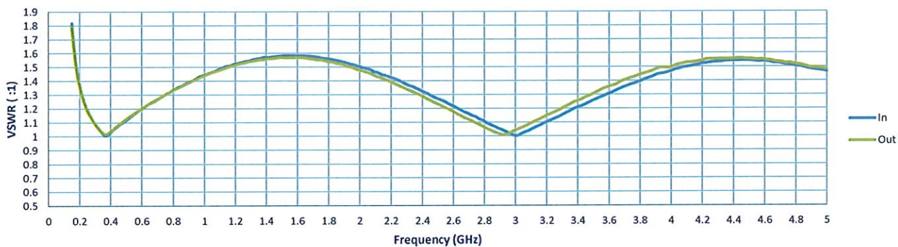
VSWR
