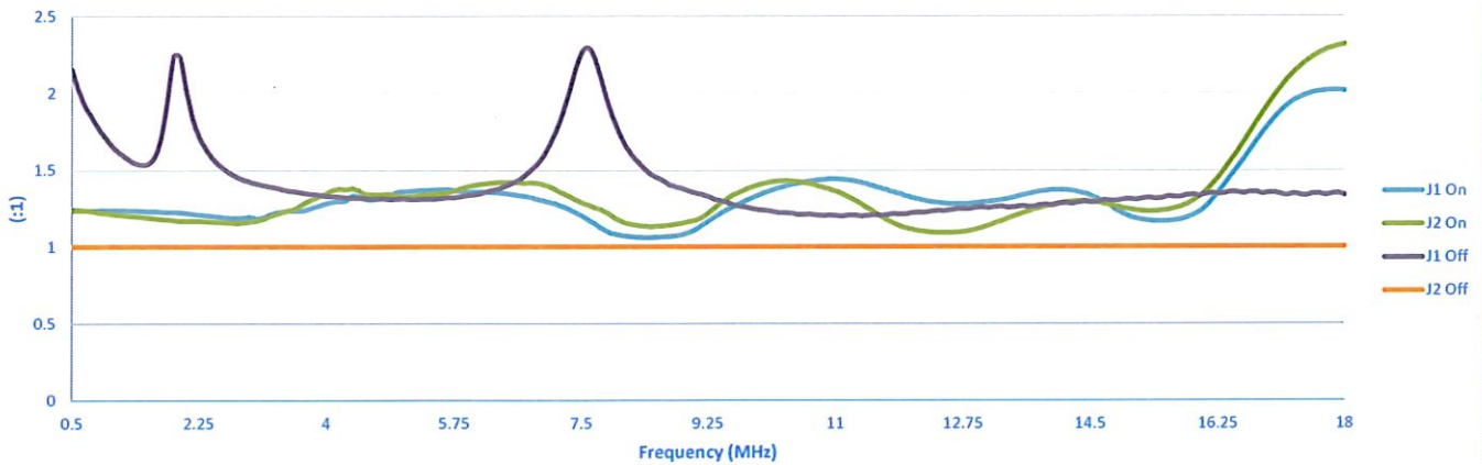
VSWR
