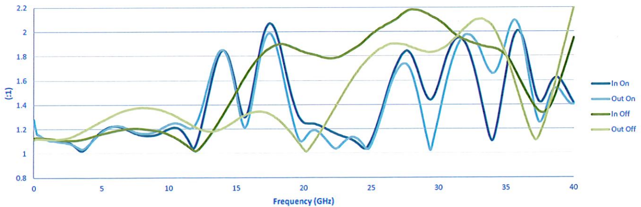
VSWR
