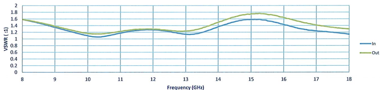
VSWR
