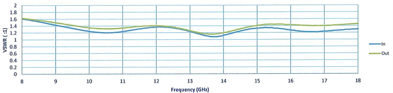
VSWR
