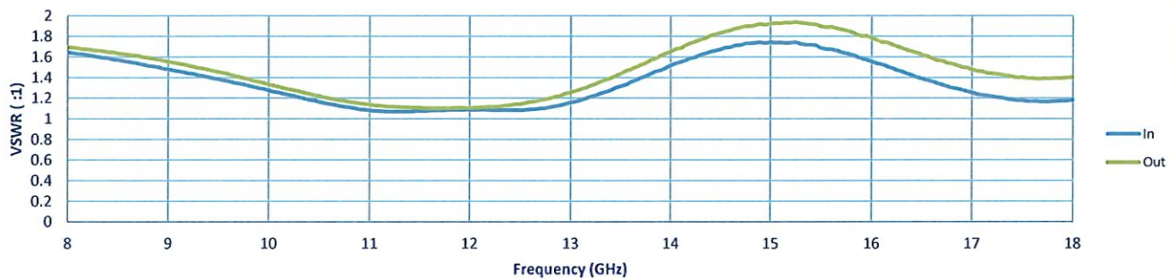
VSWR
