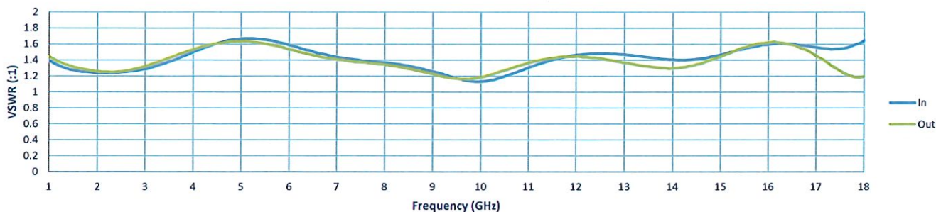
VSWR
