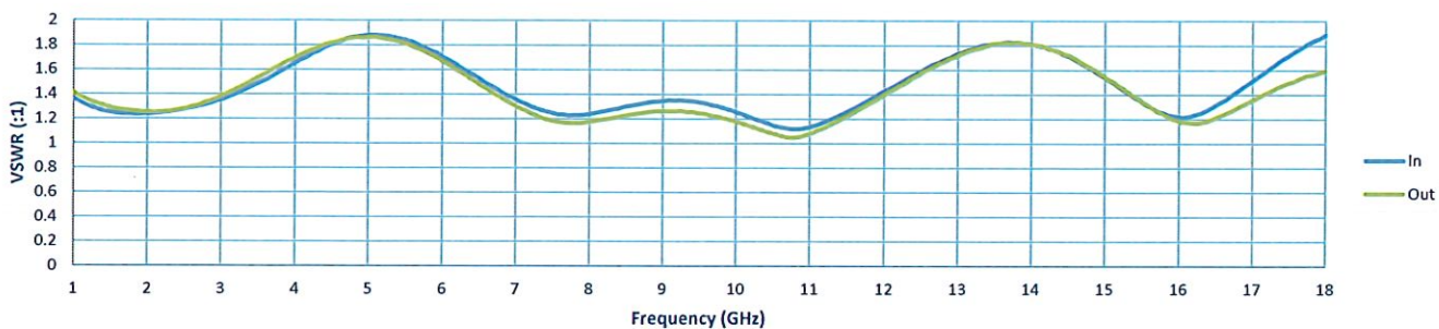
VSWR
