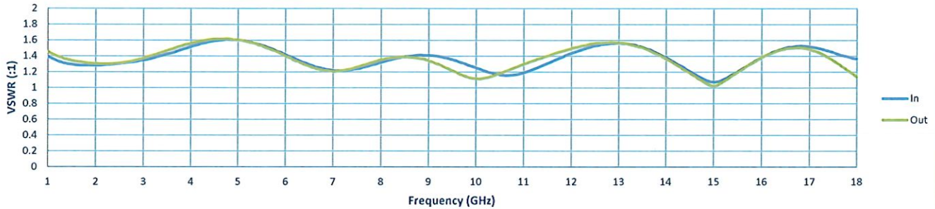
VSWR
