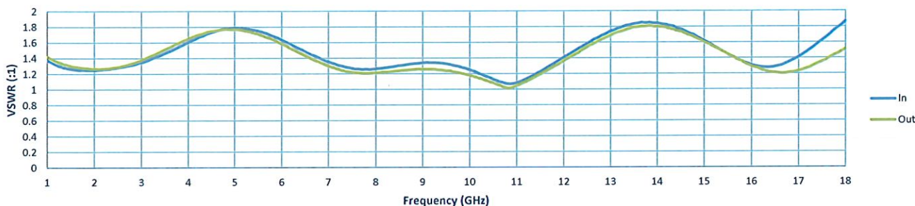
VSWR
