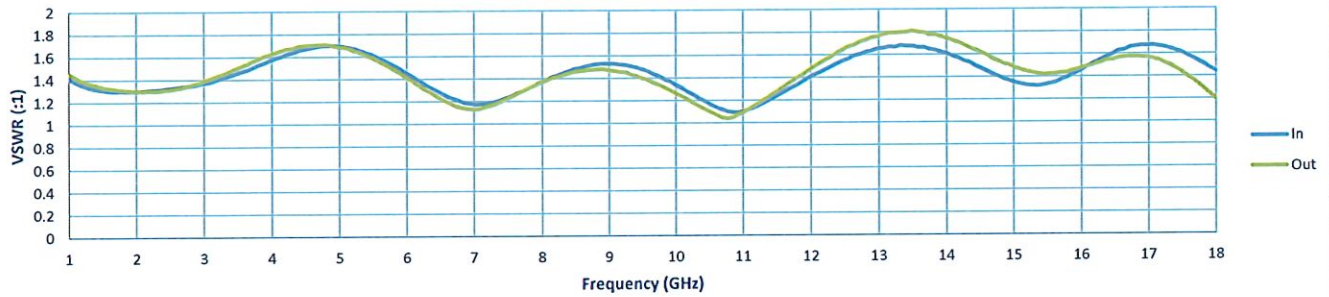
VSWR
