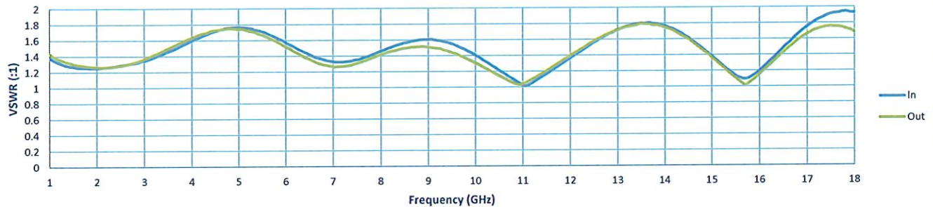
VSWR
