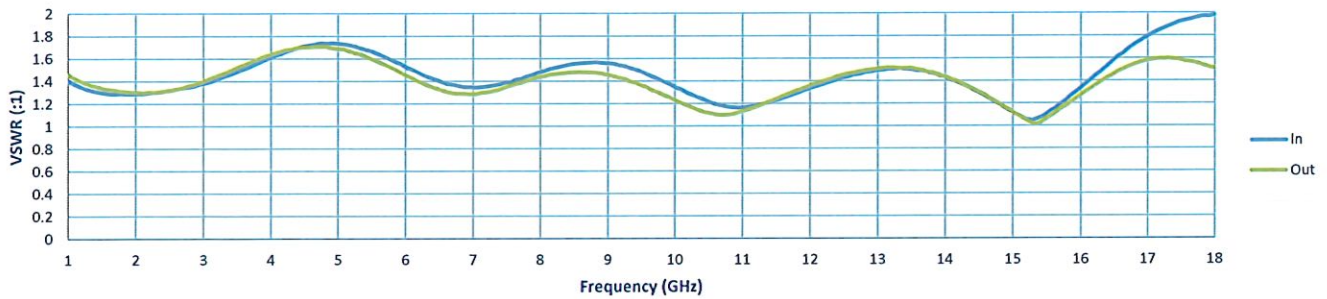
VSWR
