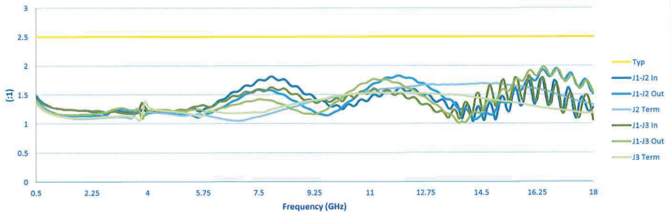
VSWR
