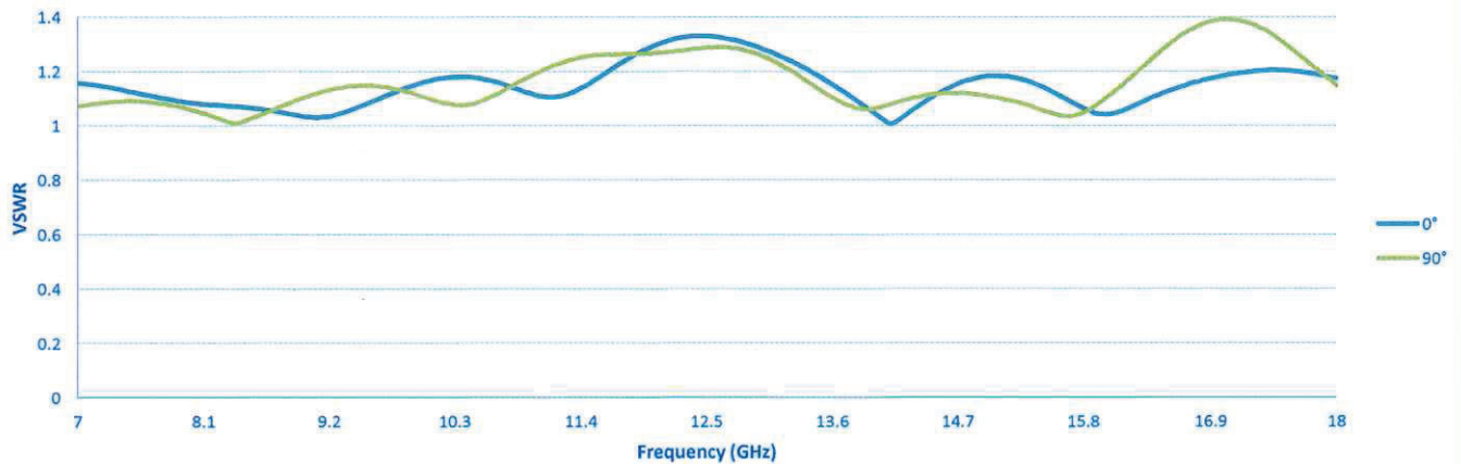
VSWR
