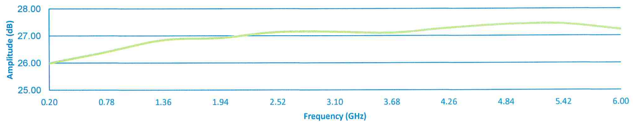
OP1dB
