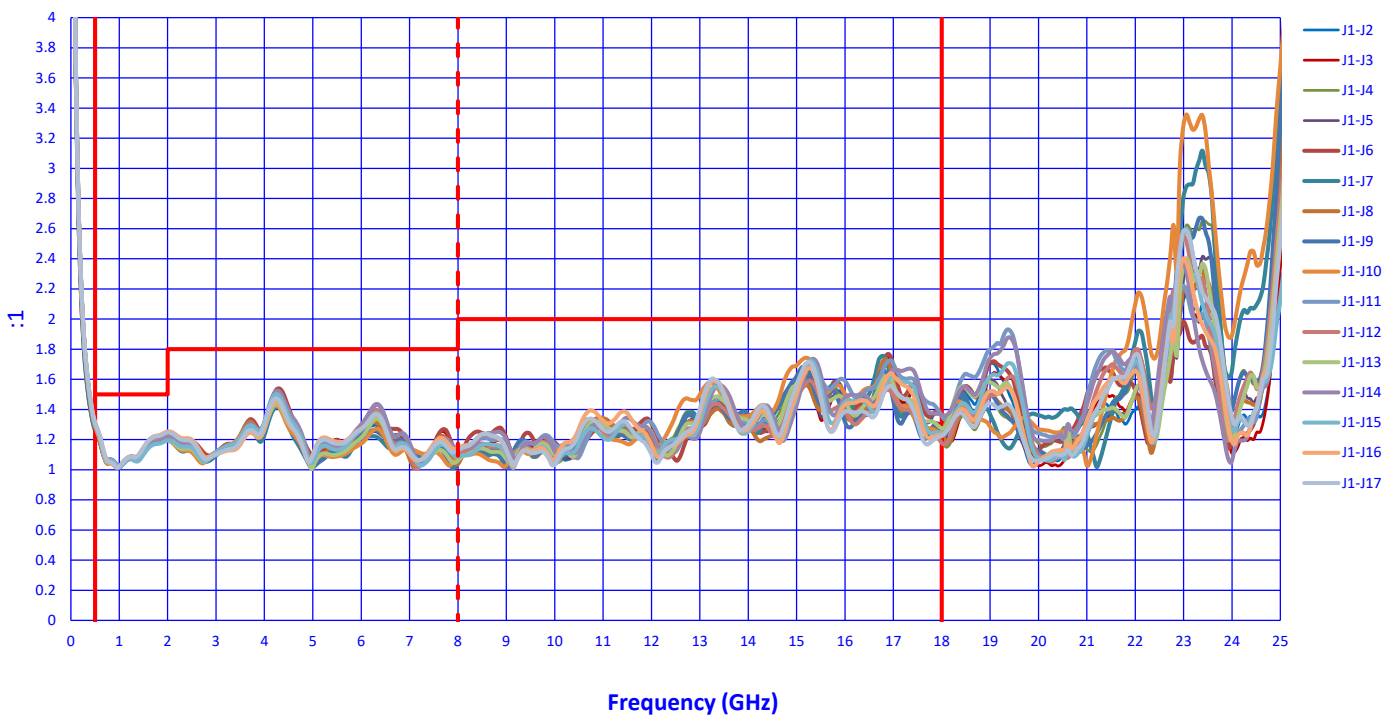
VSWR OUT (-55°C)
