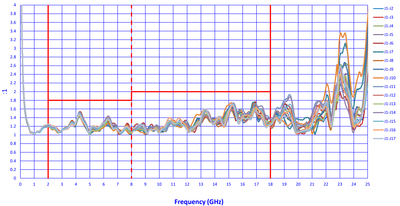
VSWR OUT (-55°C)
