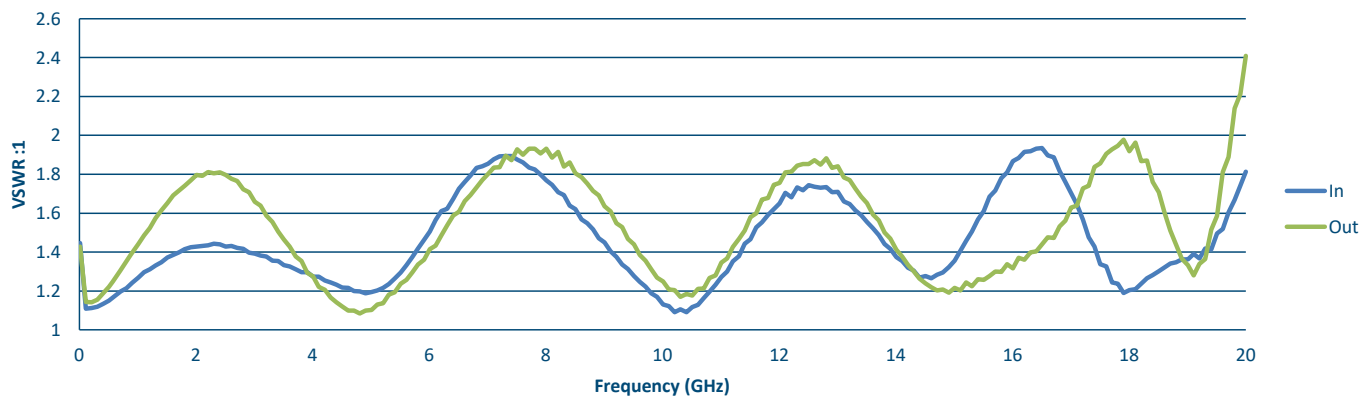
VSWR
