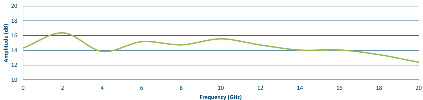
OP1dB
